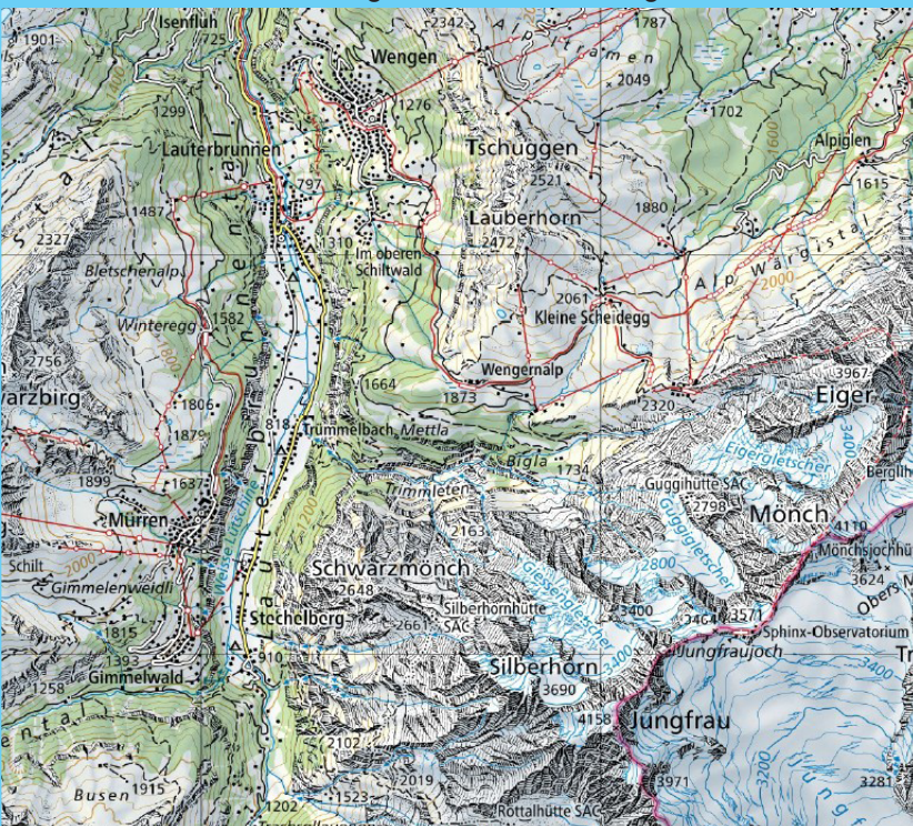
Abb. 2: Karte Lauterbrunnental
